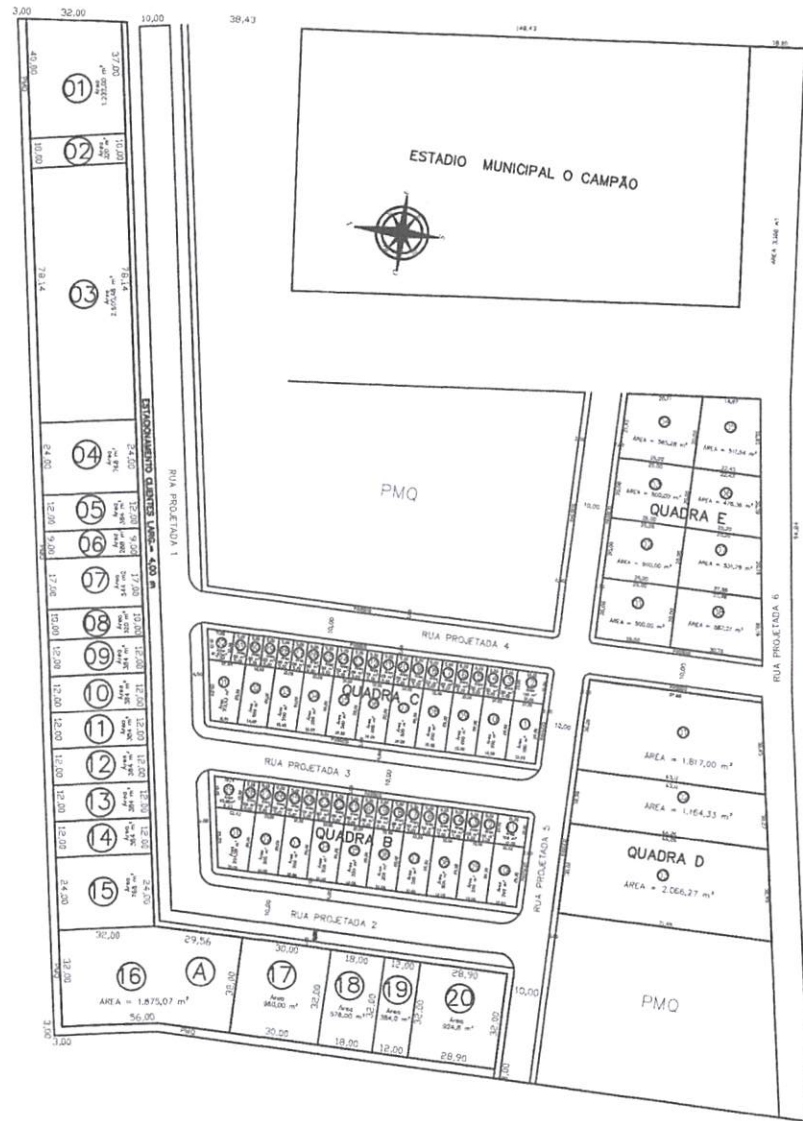
1 PLANTA BAIXA
